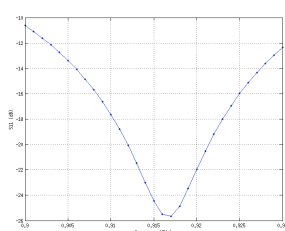
VSWR
