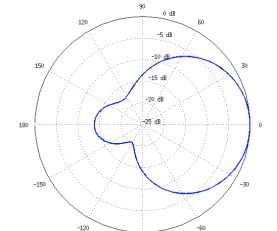
V-Pol Elevation
