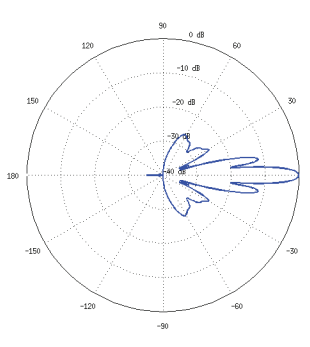
H-Plane
