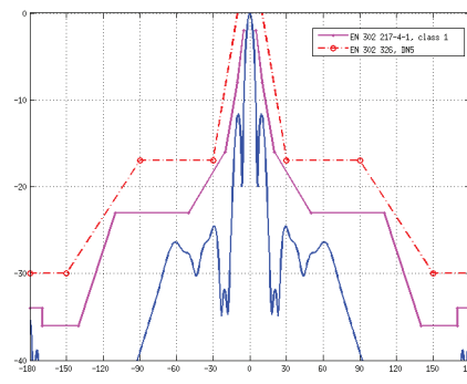
H-Plane Specs
