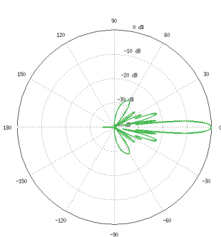
H-Plane
