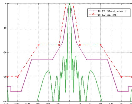
H-Plane Specs
